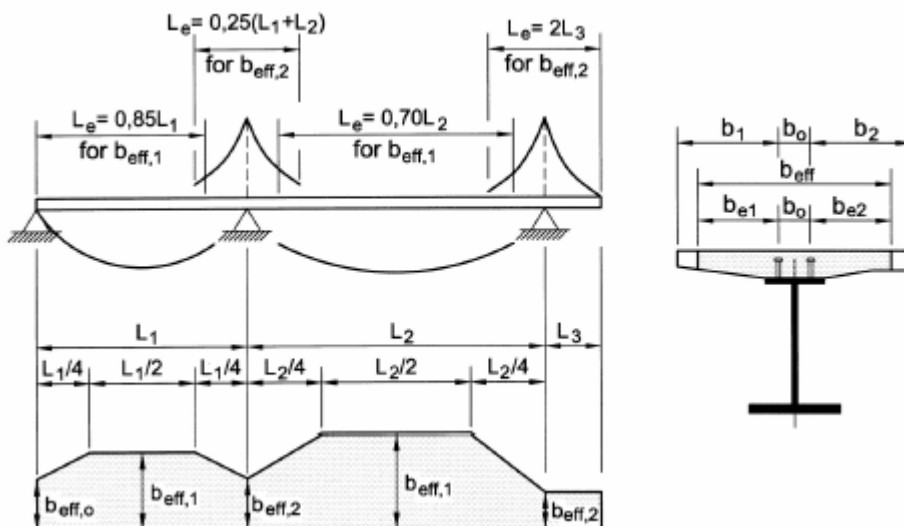
Figura 4.3.2 - Larghezza efficace, b_{\text{eff}} , e luci equivalenti, L_e , per le travi continue. (figura in italiano)
