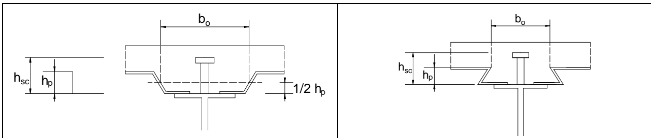
Figura 4.3.4 Disposizione della lamiera grecata rispetto al profilo in acciaio.
