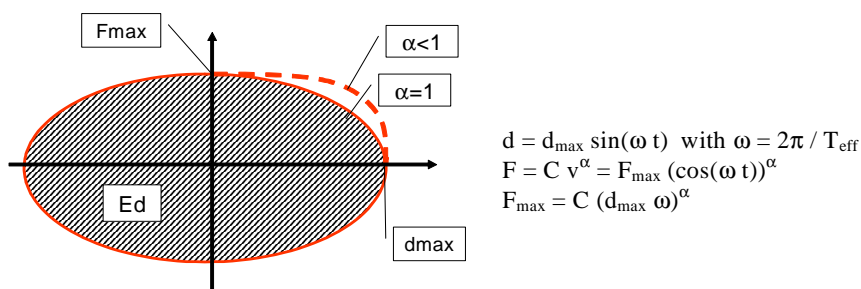
Figura 11.9.2 – Dispositivi a comportamento viscoso
